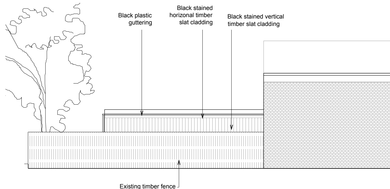
C 1:100 Elevation
