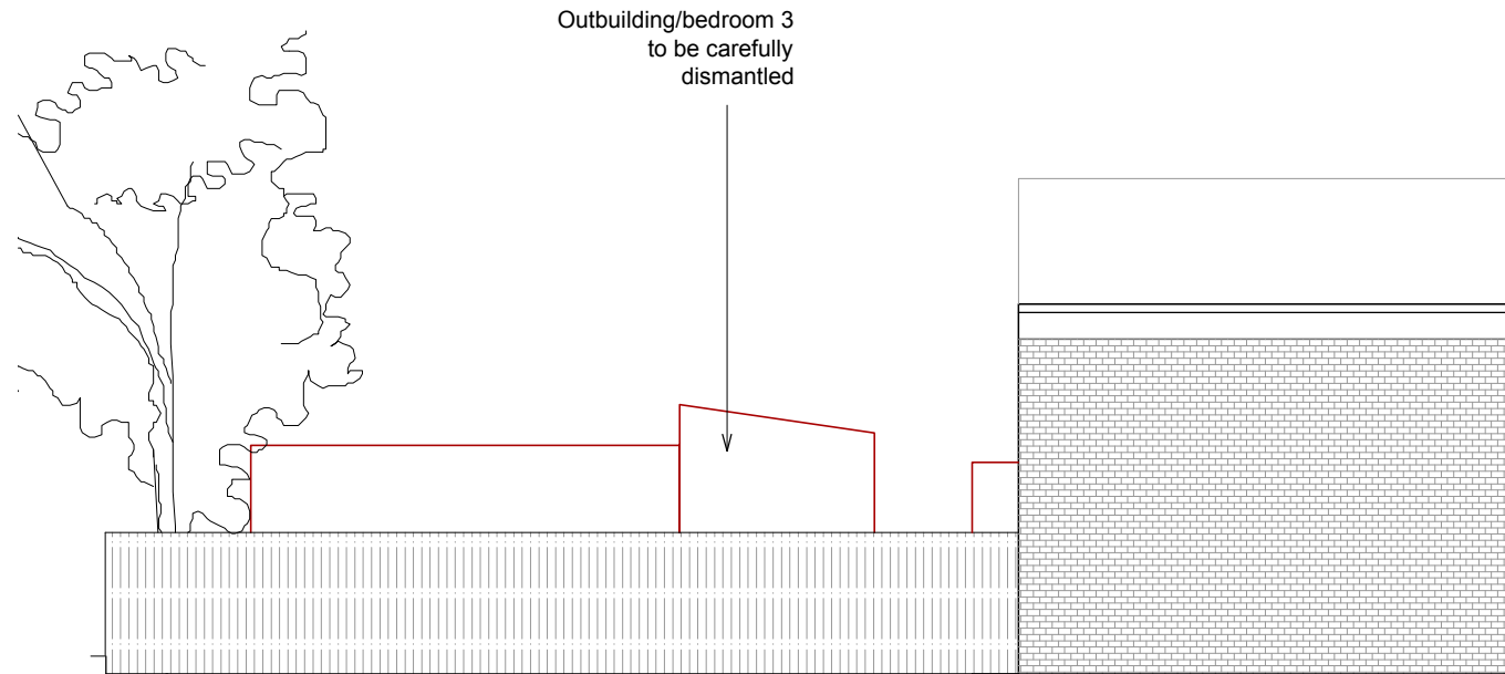
C 1:100 Elevation
