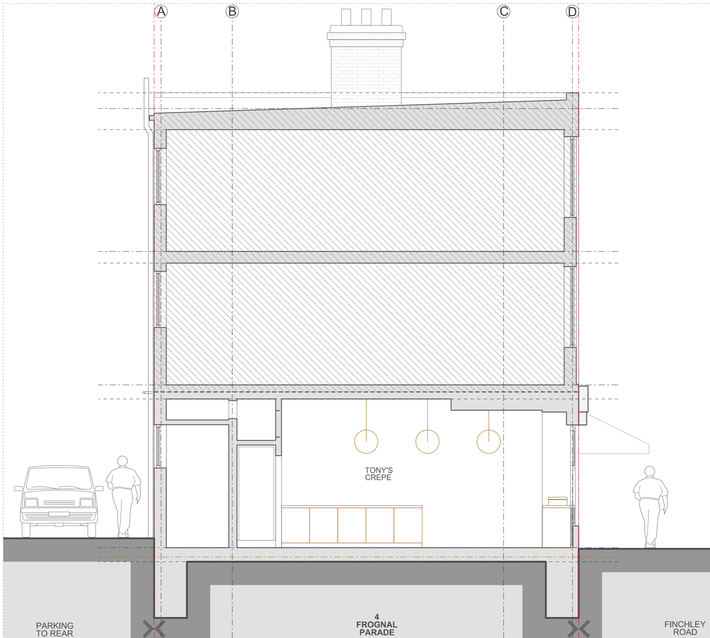
SECTION A-A - EXISTING SCALE 1:50 @ A3
