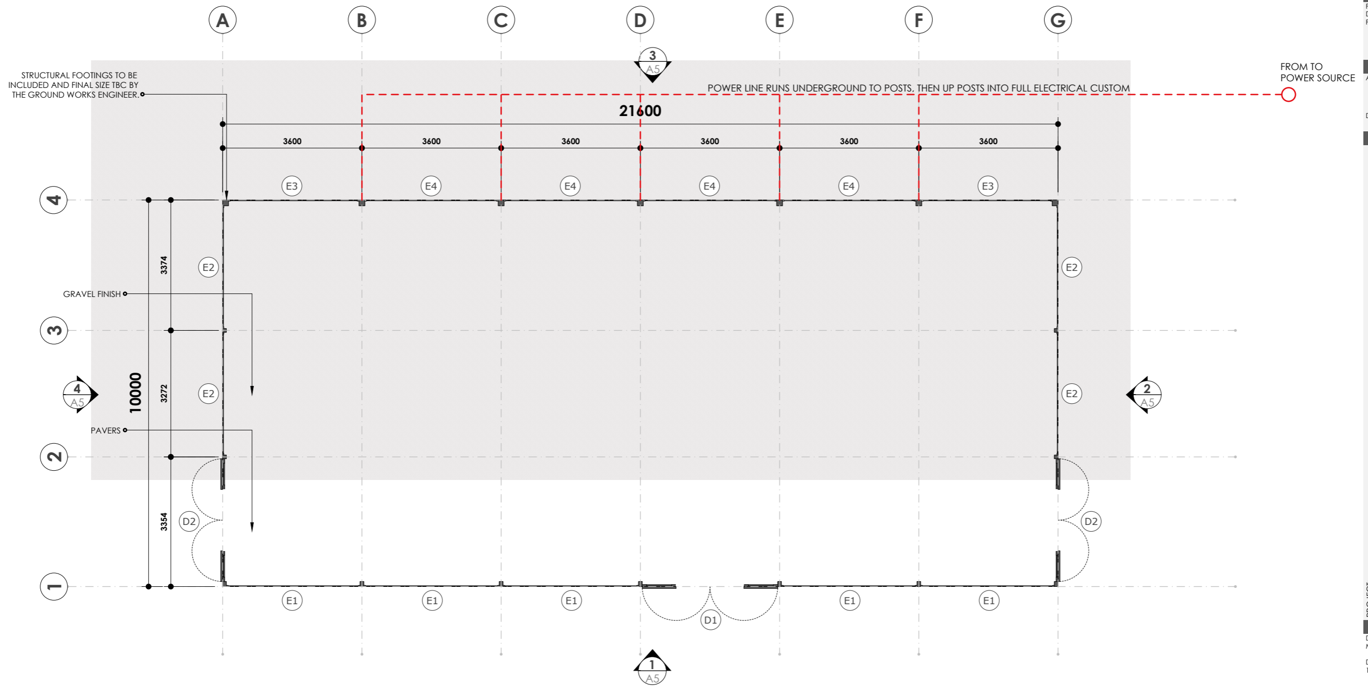
FLOOR PLAN SCALE: 1:50 M
