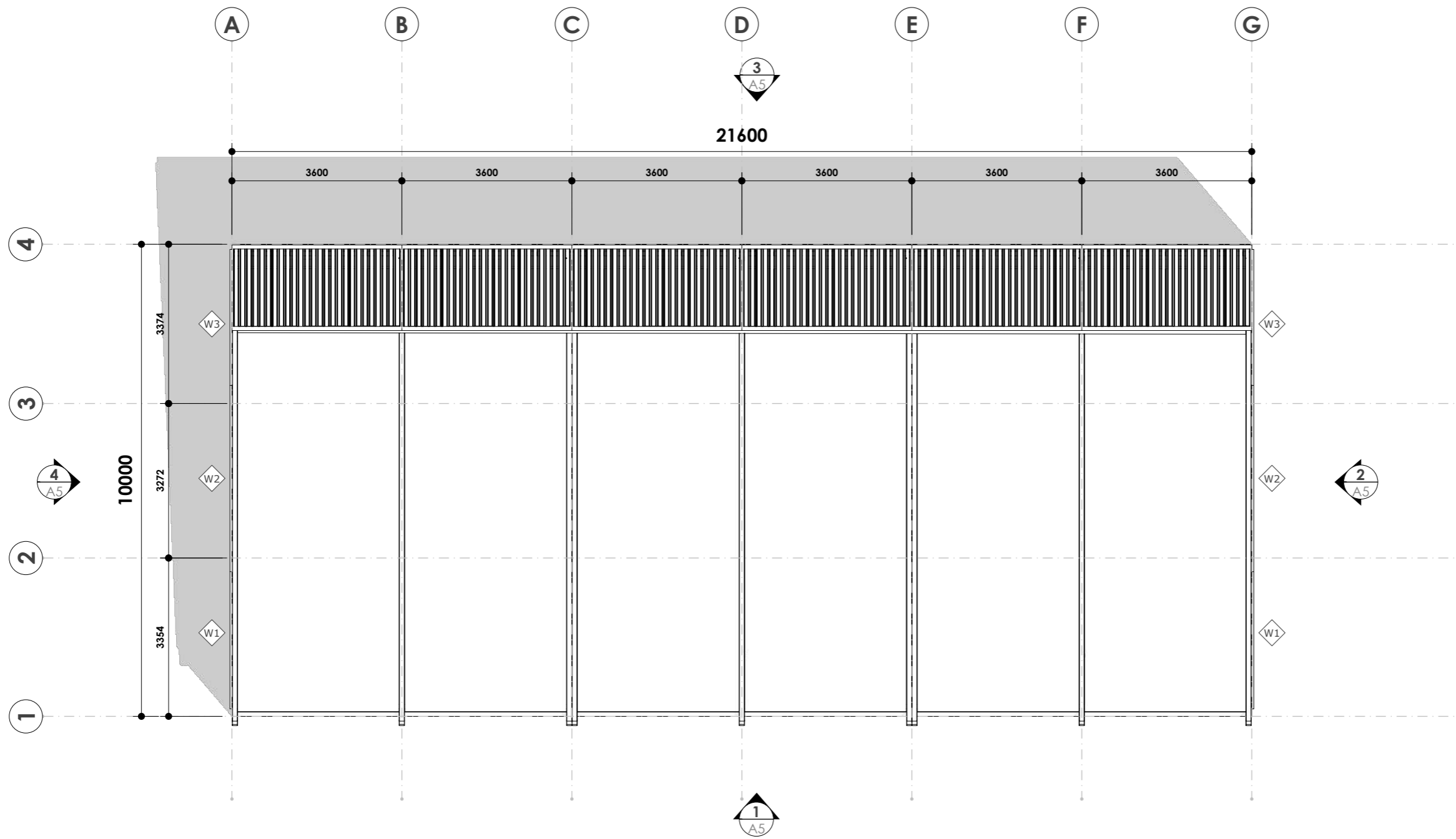
1 A4 ROOF PLAN SCALE: 1:50 M
