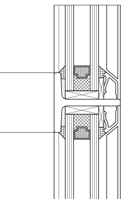
OPTIONAL GLAZING BAR
