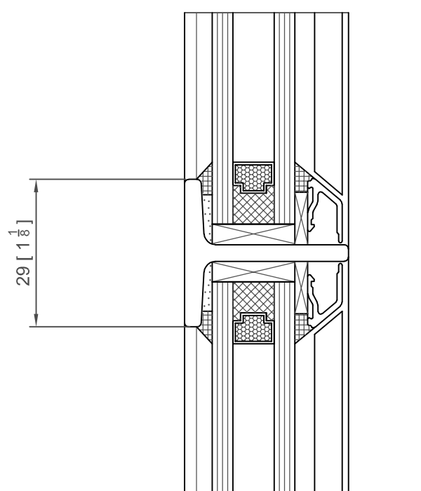
OPTIONAL GLAZING BAR
