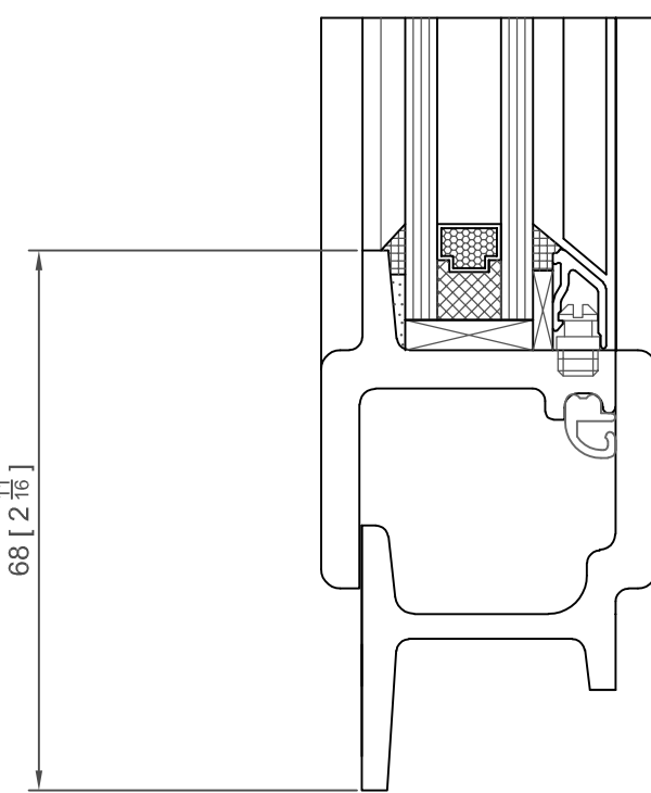
UNEQUAL LEG OPTION SHOWN
