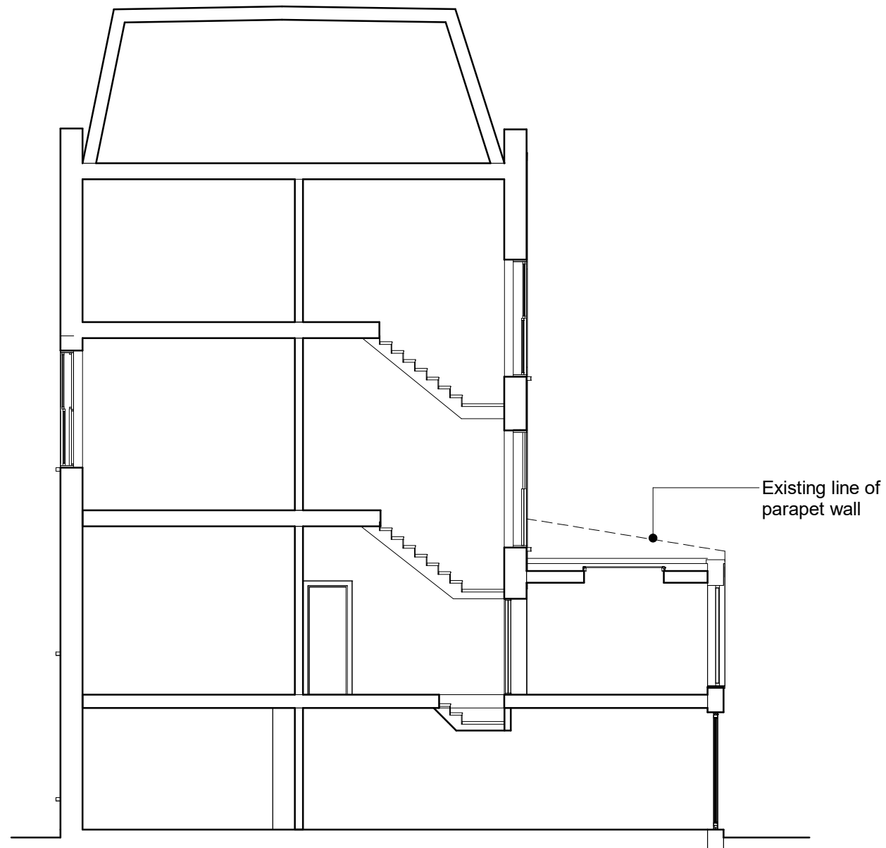
01 Section A-A 1 : 100
