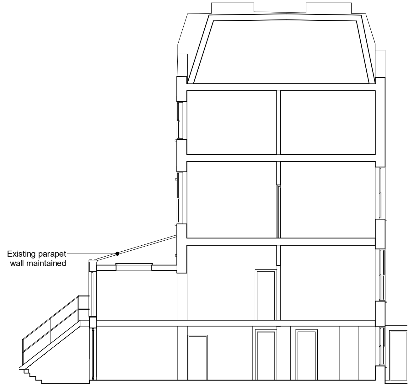
02 Section B-B 1 : 100
